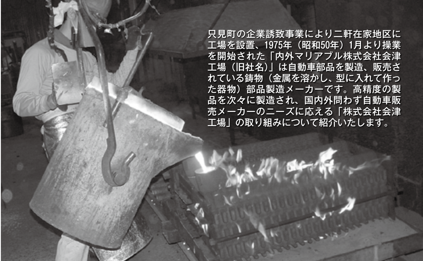
▲Hプロセス工法による製品の製造（鋳込み）
