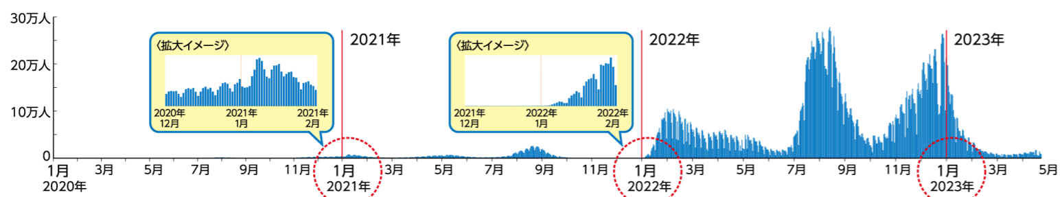
〈日本における新型コロナウイルス変異株の変遷イメージ〉
